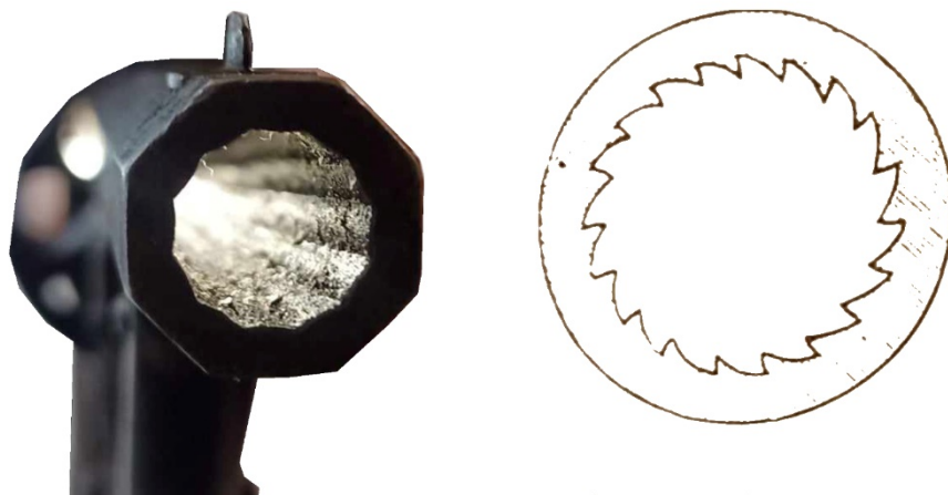
Figura 11. Țeava și profilul ghinturilor/ The barrel and the profile of the rifling
